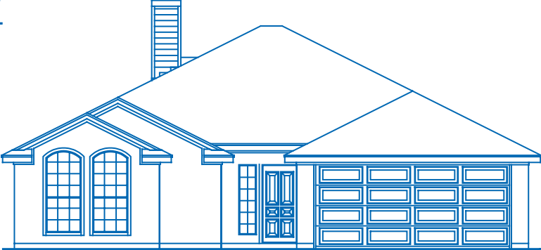
ELEVATION "C"
